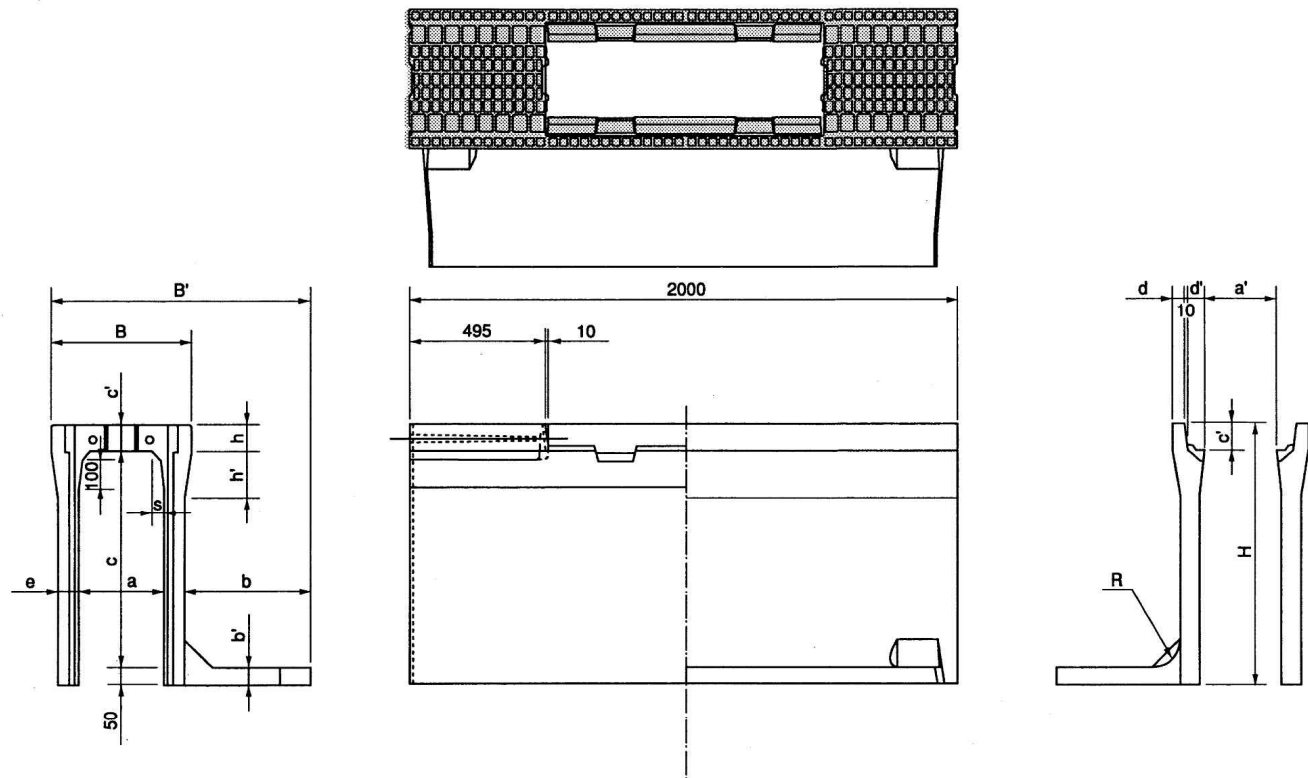
本体標準図 [ 縦断用 ]
